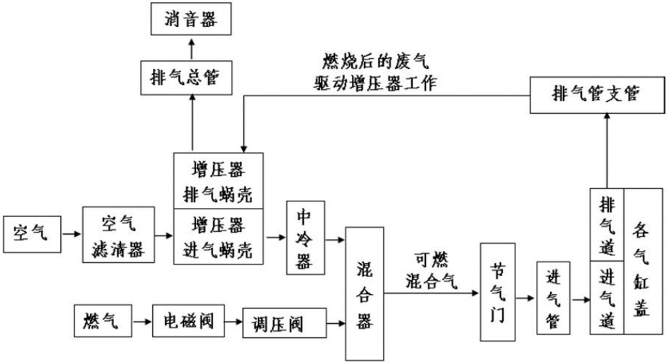
图3 伴生天然气发动机进、排气系统工作流程图
