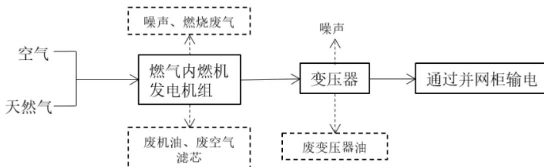
图2 运营期工艺流程及产污节点示意图
