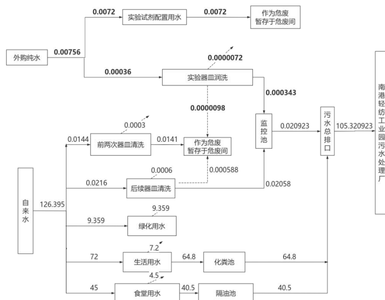
图 2-1 本项目水平衡图 单位: m 3 /d
