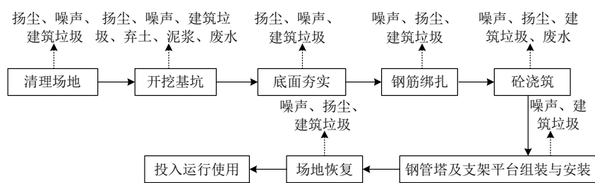
图 2-4 新建终端角钢塔（带电缆平台）施工工艺流程图
