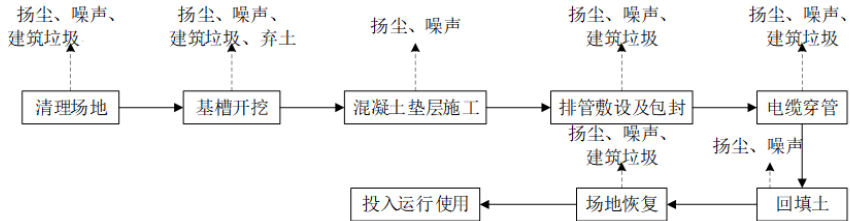
图 2-5 电缆排管施工工艺流程及产污节点图
