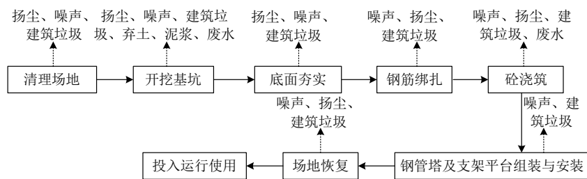
图 2-4 新建电缆终端钢管塔（带电缆平台）施工工艺流程图
