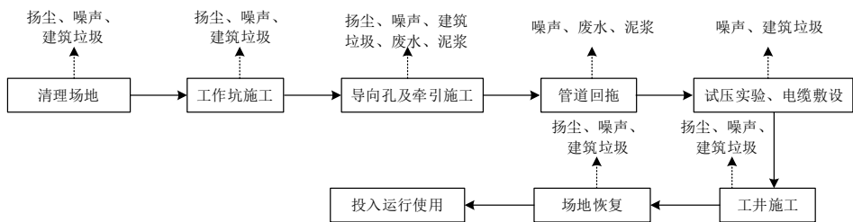
图 2-5 拉管敷设施工工艺流程及产污节点图
