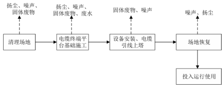
图 2-5 电缆终端平台施工期工艺流程图
