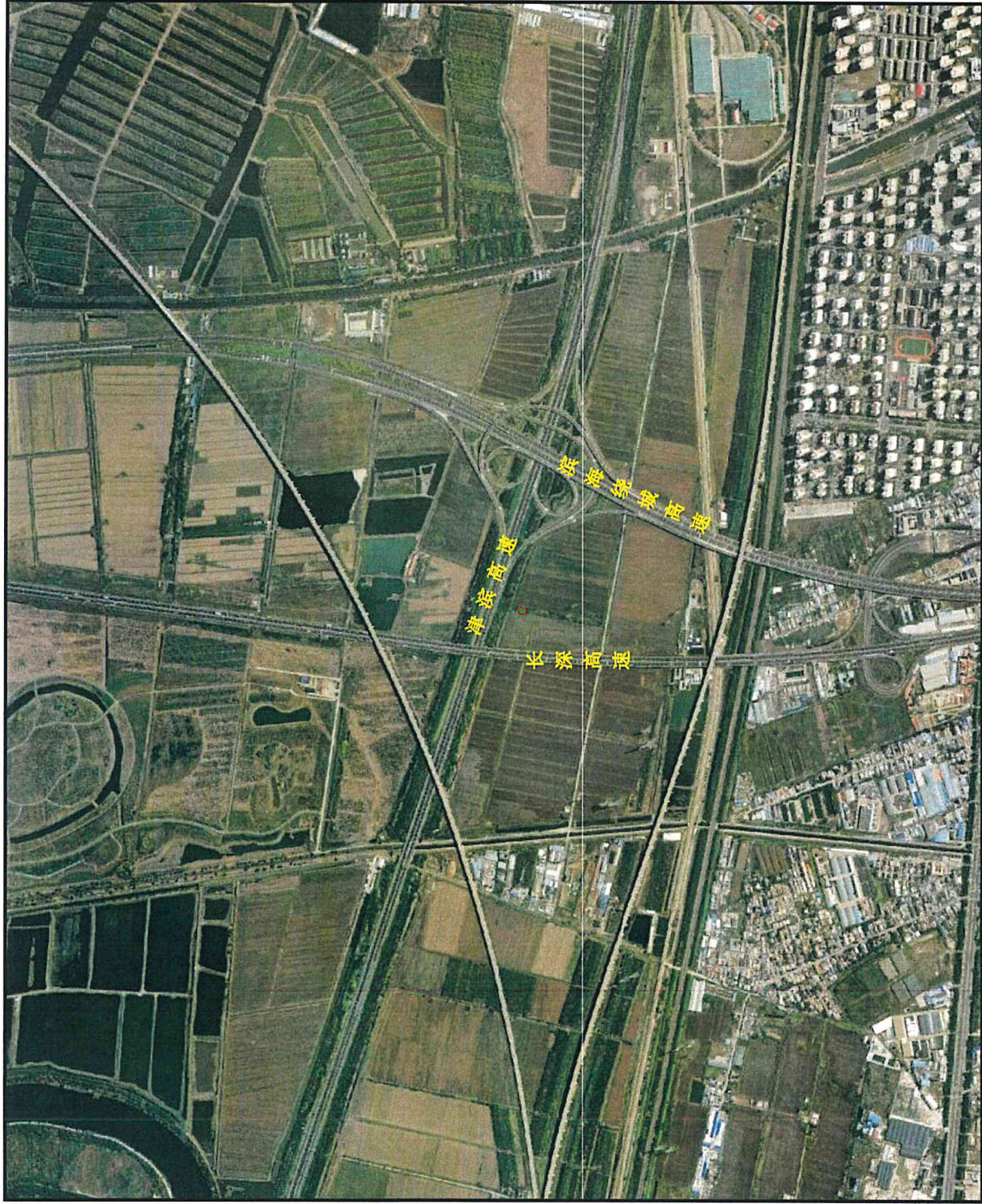
附图1 220千伏滨中一二线、滨幸一、滨幸一二线迁改工程拟使用林地位置图(永久)
